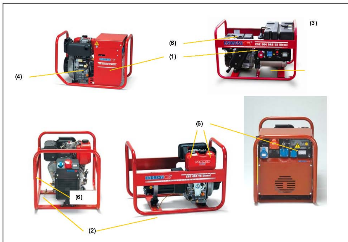
Рис. 2.1: Обозначения на генераторе
