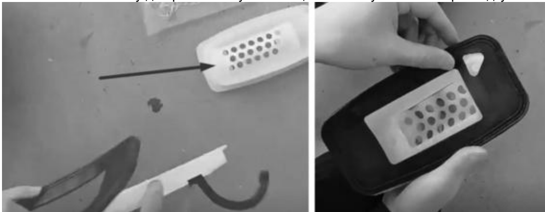
Рисунок 17 – Сборка пластины для работы с сухими веществами
