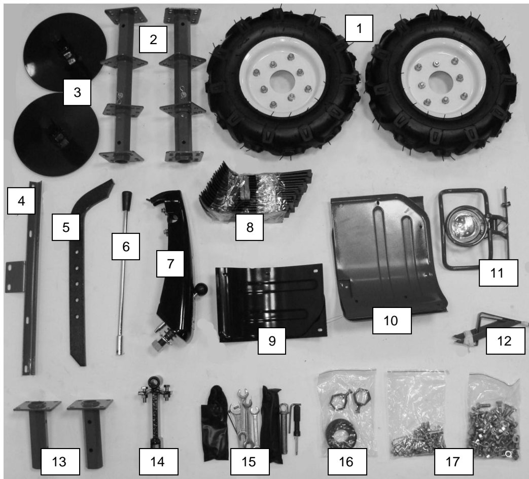
Рис. 2. Комплект поставки.
