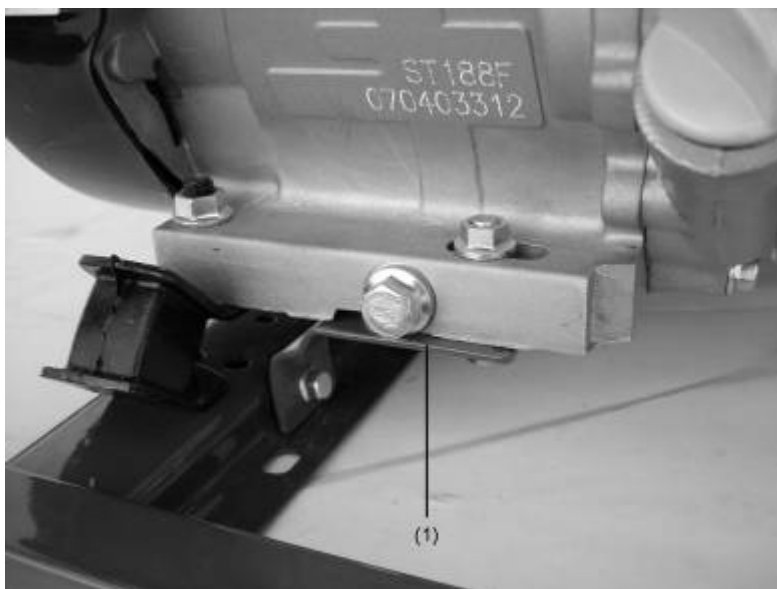
Рис. 4.1: транспортировочных креплений
