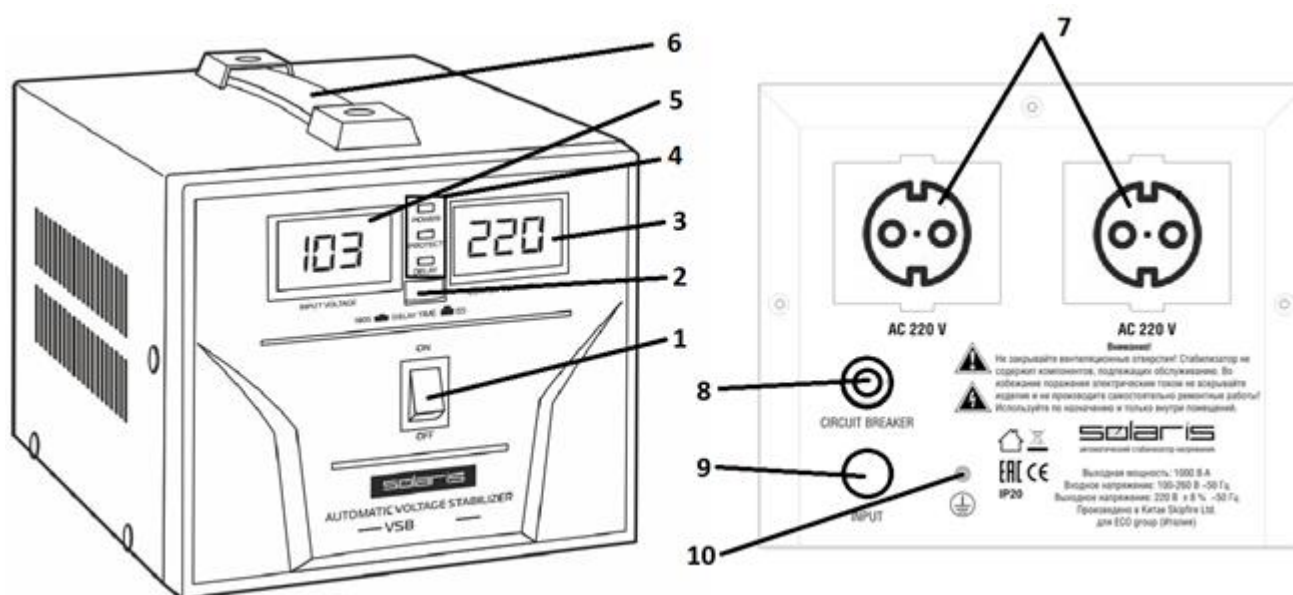
Рисунок 1 – Устройство стабилизатора
