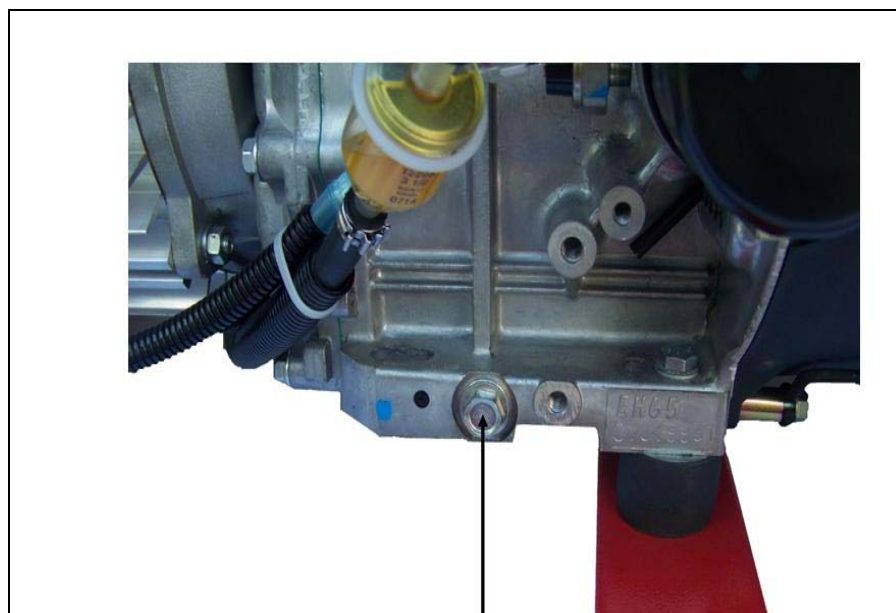
Рис. 5-3: Замен масла
