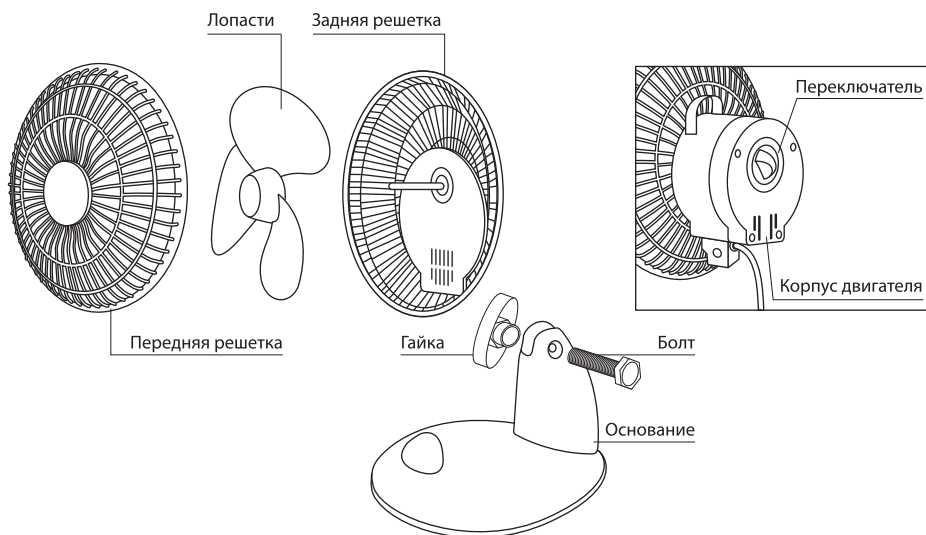
Рисунок 1. Конструкция вентилятора
