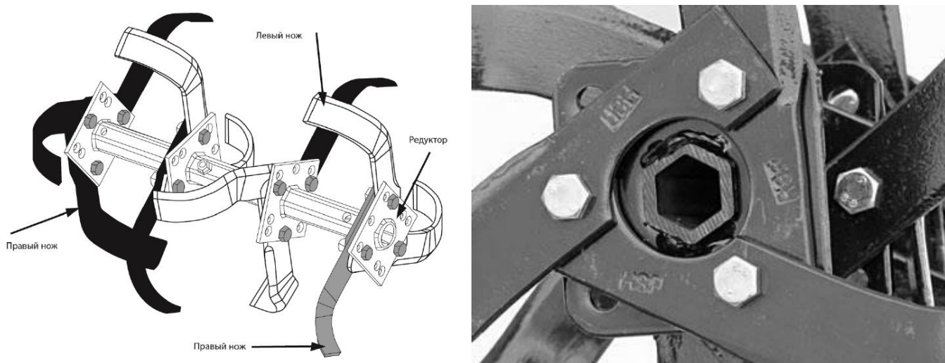
Рисунок 2 – Сборка фрез
