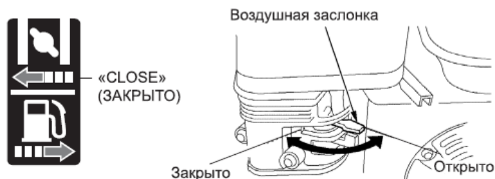
Рисунок 9 – Воздушная заслонка
