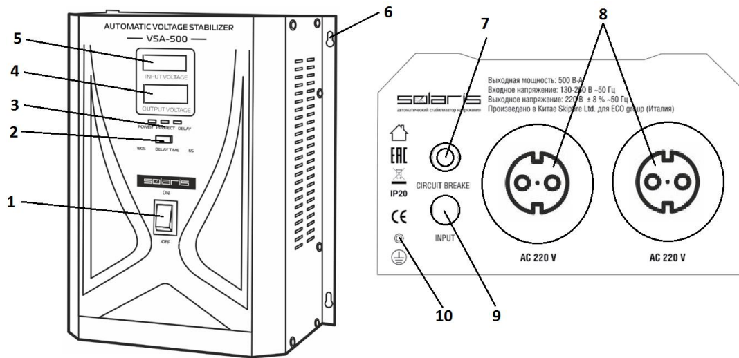
Рисунок 1 – Устройство стабилизатора
