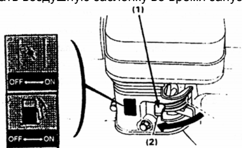
(1) Переключатель воздушной заслонки. (2) Положение “Закрыто”.
