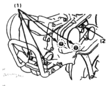
(1) установочные болты двигателя. (2) крепежный болт двигателя.
