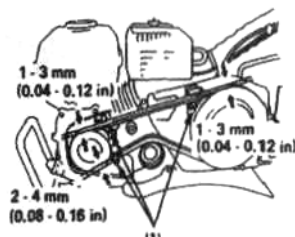
(1) стопорный механизм ремня.
