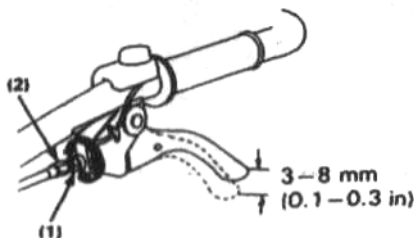
(1) стопорная гайка. (2) регулировочный болт.
