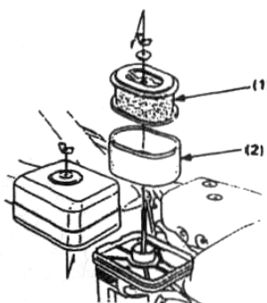
(1) бумажный элемент. (2) пористорезиновый элемент.
