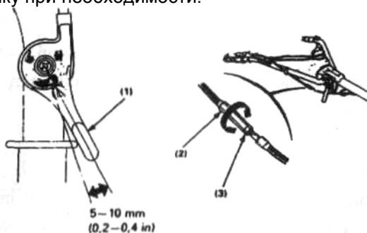
(1) рычаг дроссельной заслонки. (2) регулировочная гайка. (3) стопорная гайка.
