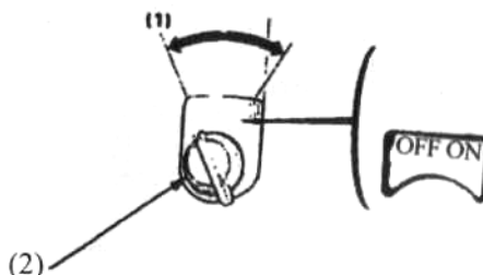
(1) положение "выключено" (OFF). (2) переключатель двигателя.
