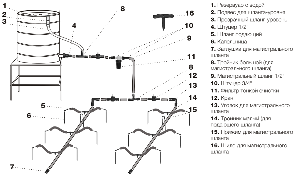
Рис. 1 Принципиальная схема сборки системы для капельного полива
