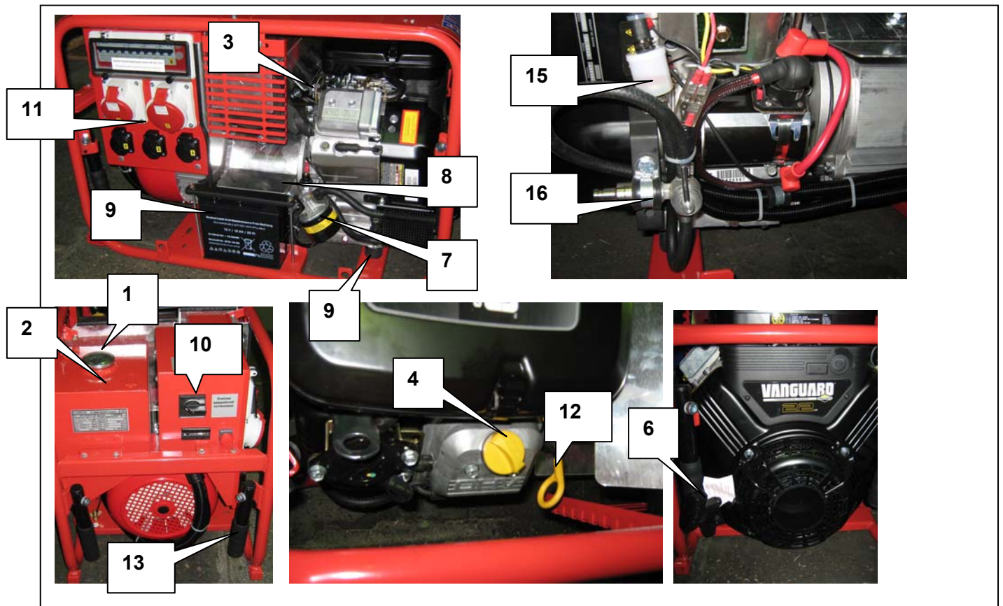
Рис 3.1. Элементы электростанции
