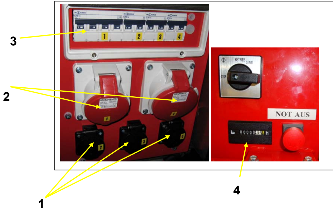
Рис. 4.4: Подключение потребителей
