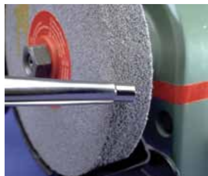
Промежуточное шлифование
