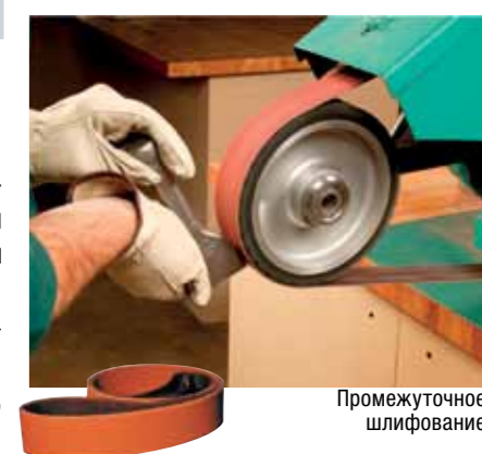
Шлифовка валов
