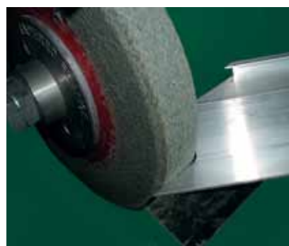
Удаление заусенцев
