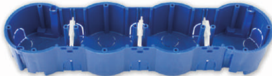
KE-503* Коробка четырехместная для крепления выключателей и розеток Размер коробки: 278x66x47,4 мм
