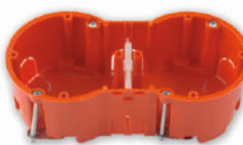
KE-504* Коробка двухместная для крепления выключателей и розеток Размер коробки: 136x66x47,4 мм
