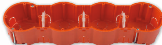
KE-506* Коробка четырехместная для крепления выключателей и розеток Размер коробки: 278x66x47,4 мм
